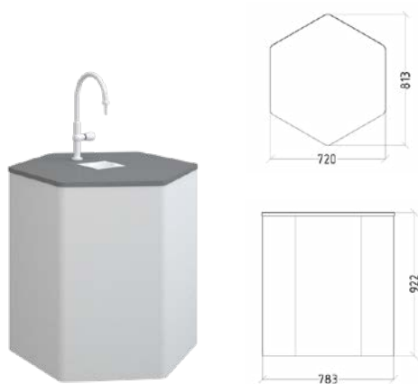
ТУМБА СЕРВИСНАЯ ХИМИЧЕСКАЯ СТАЦИОНАРНАЯ С МОЙКОЙ 813x720x922
