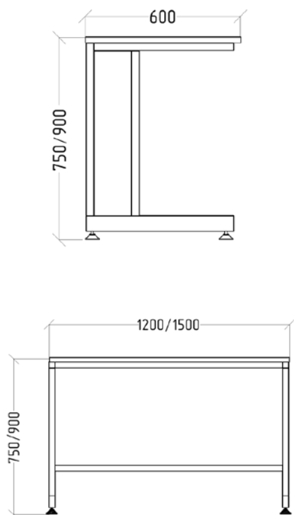
СТОЛ ЛАБОРАТОРНЫЙ
